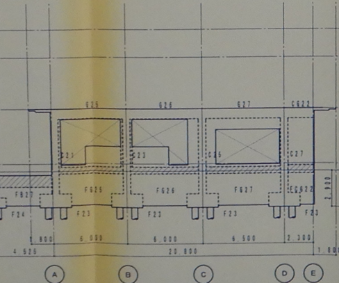
8通り軸組図 1/200
