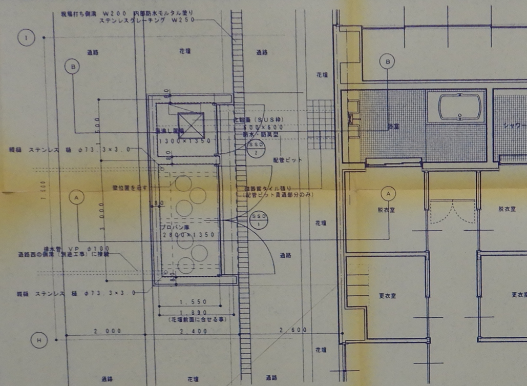
プロパン庫・湯沸器置場 平面図 1 / 50
