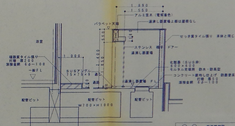
⑤—⑥ 断面詳細図 1 / 50
