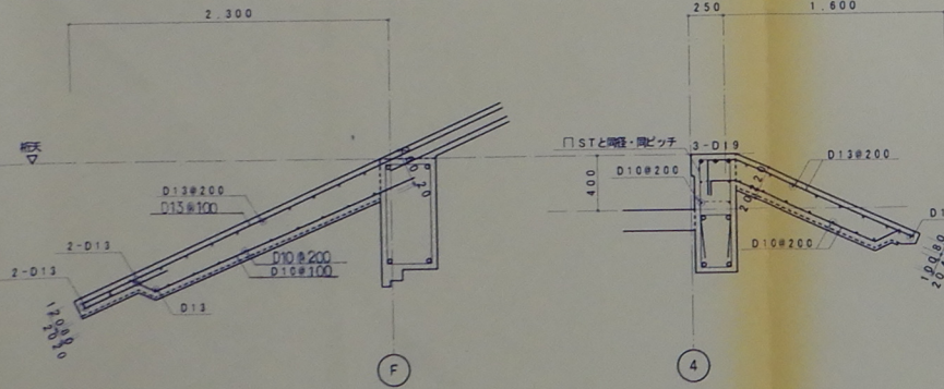
庇配筋要領 S=1/30
