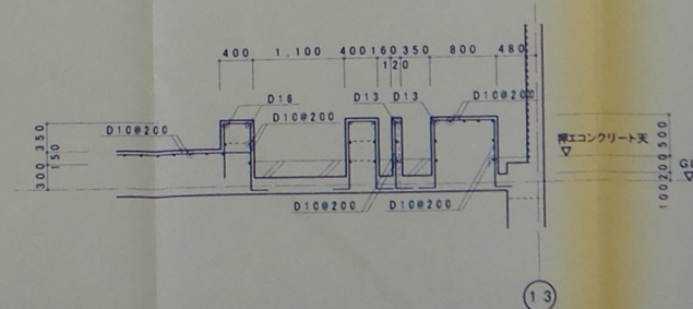
機械室内設備用基礎配筋図 S=1/50
