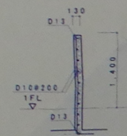
浴場洗い場立上り壁配筋図 S=1/50
