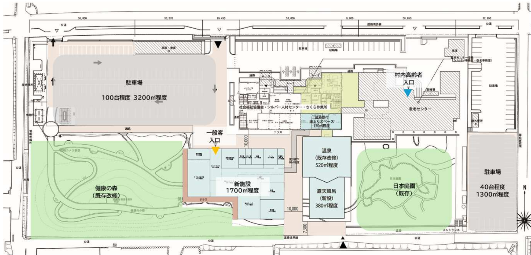
図 敷地全体の平面計画 (案)
