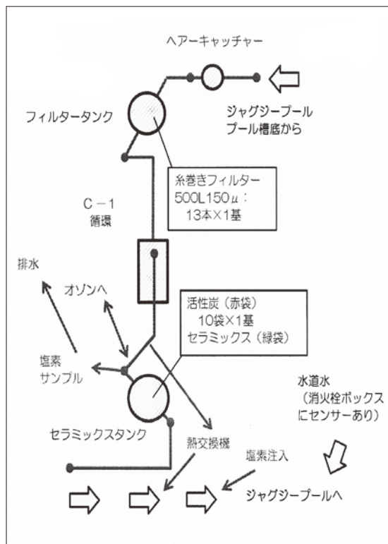
温水プール浄水設備の概要
