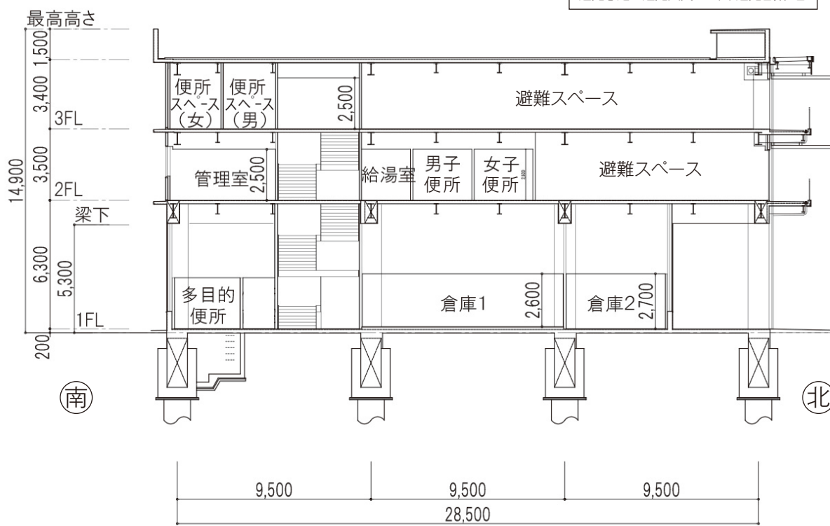
断面図
