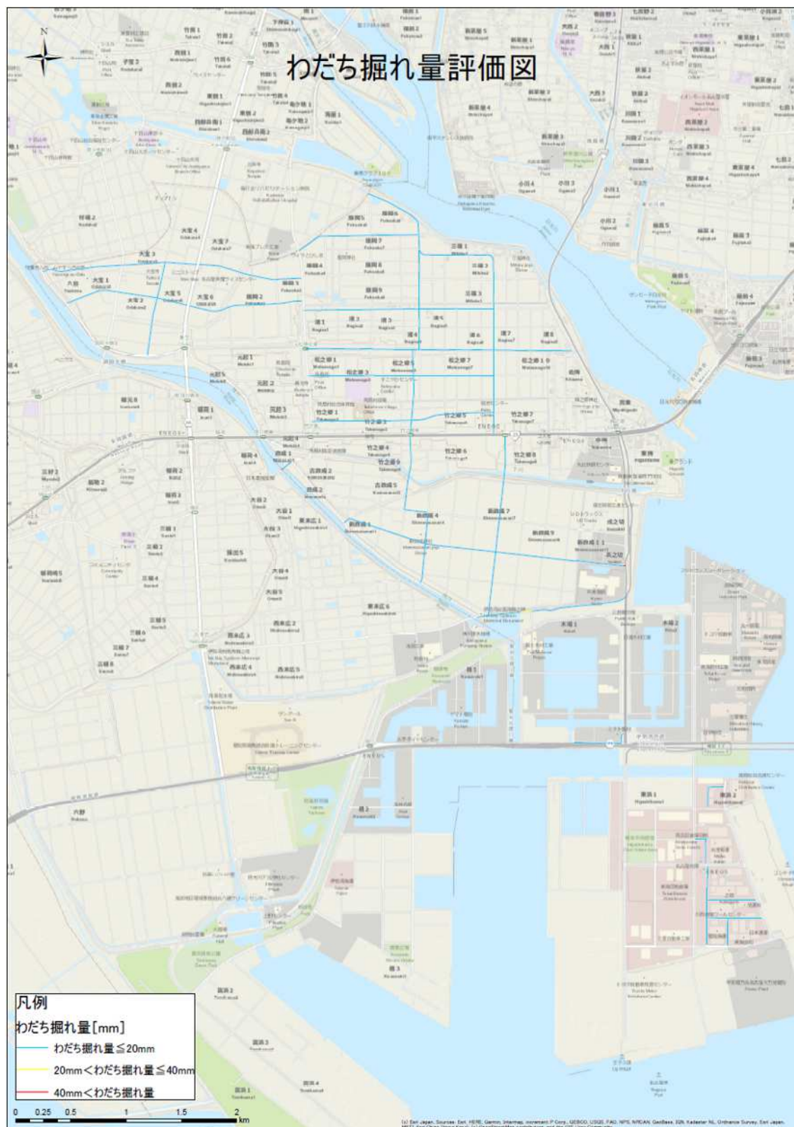
図 4 わだち掘れ評価図
