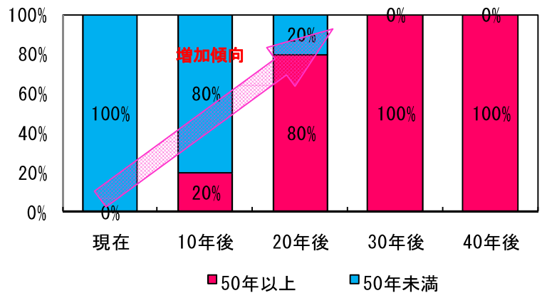
図-3.5 架設後 50 年以上の橋梁割合
