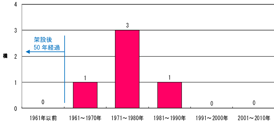
図-3.3 架設年次別の橋梁数
